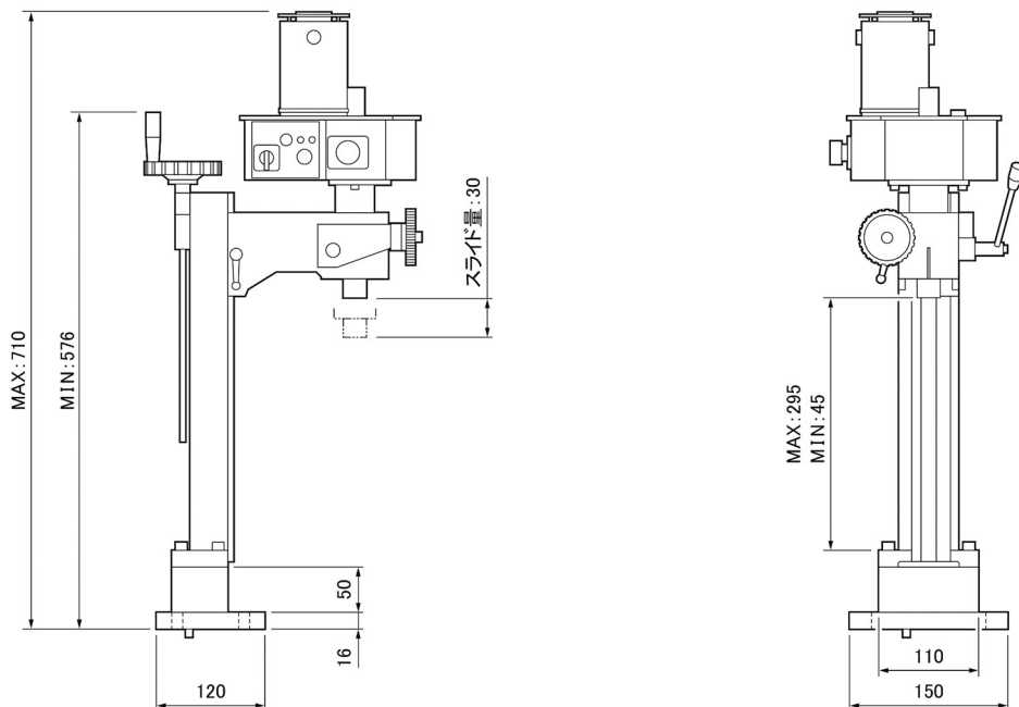
外觀2面寸法図
