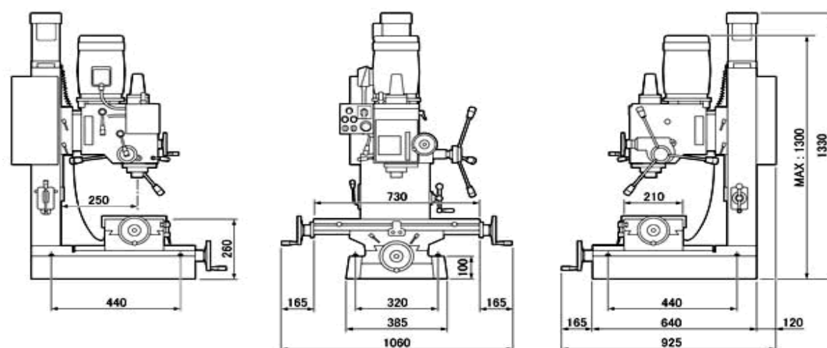
M45 小型フライス盤 (Z軸(上下)自動早送り・タッピング機構搭載) 外観3面寸法図
