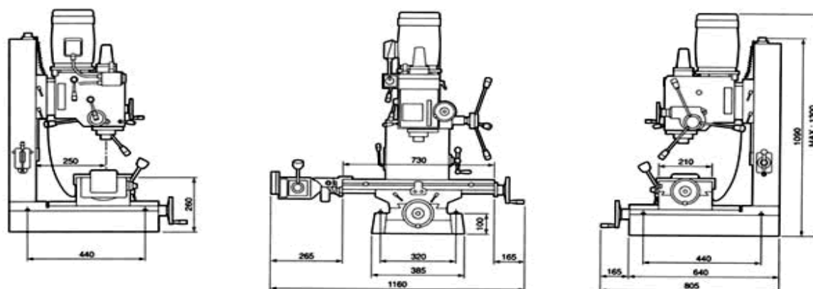
M45 小型フライス盤 (長手自動送り装置付き) 外観3面寸法図
