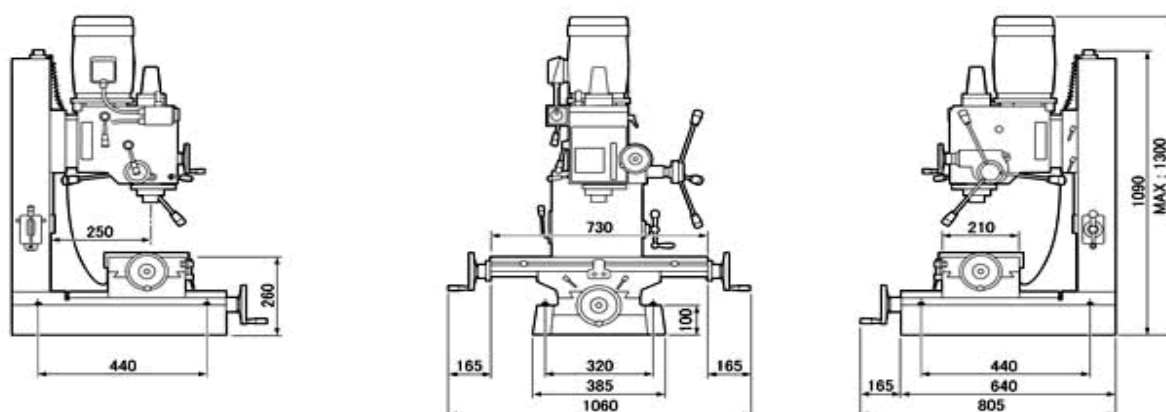
M45 小型フライス盤 外観3面寸法図
